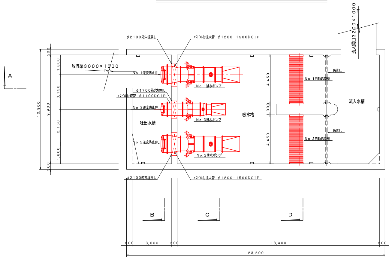
屋外 (下部) 平面図 S=1/100
