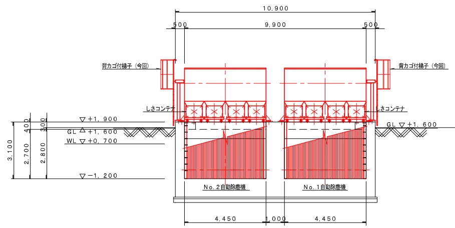
D-D 断面図 S=1/100
