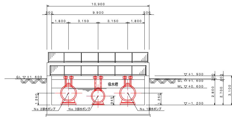
C-C 断面図 S=1/100
